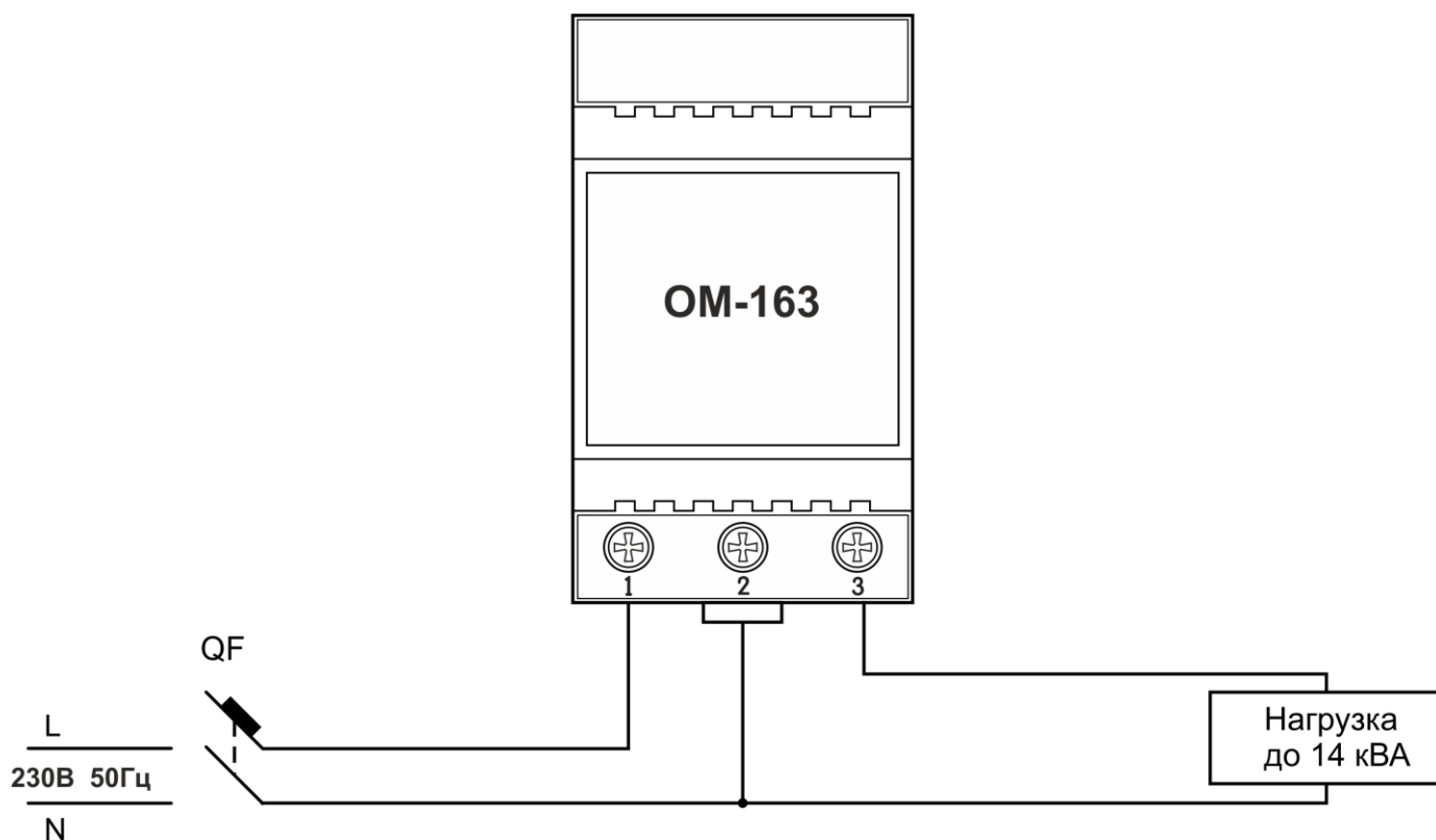
Рисунок 2 – Схема подключения изделия
