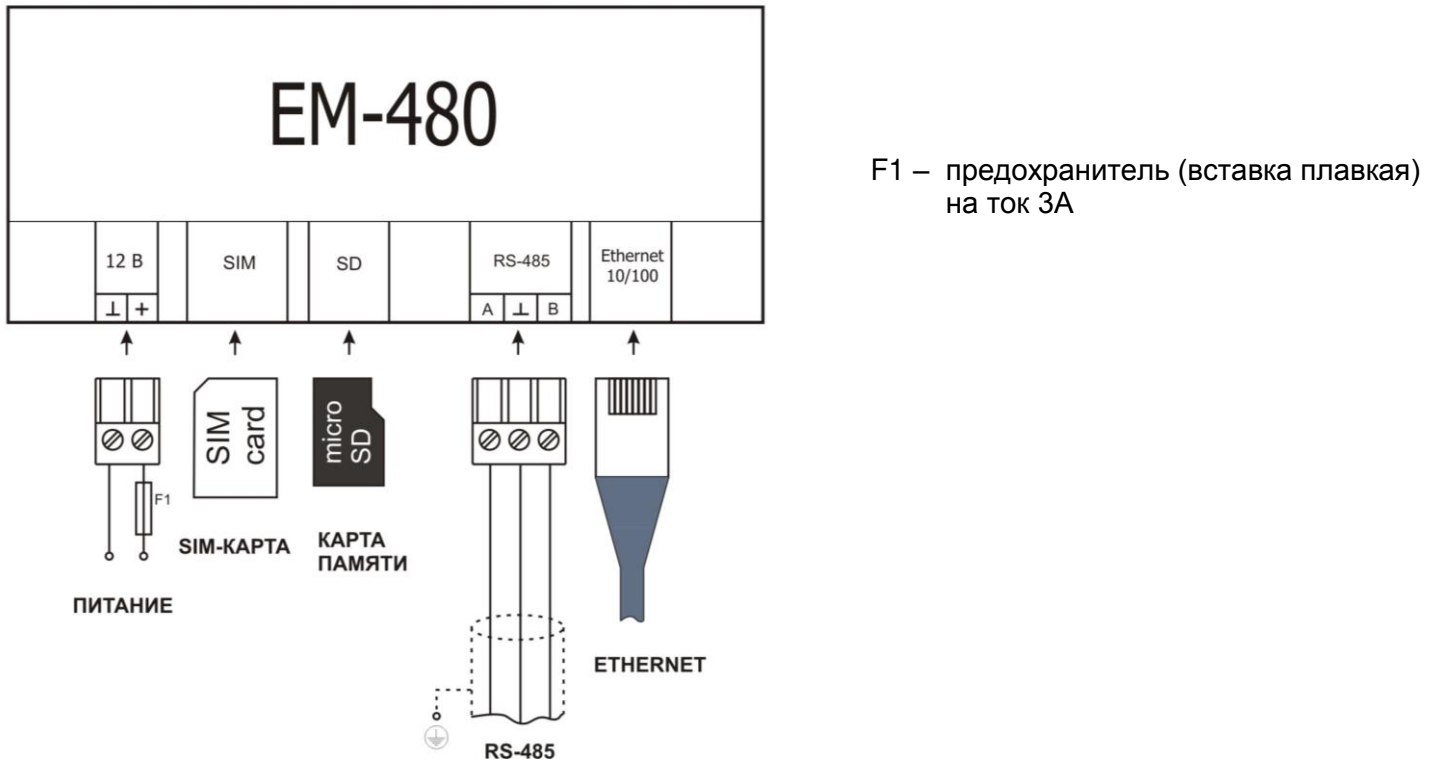
Рисунок 5.1 – Подключение изделия
