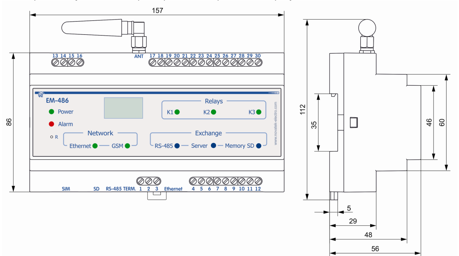
Рисунок 1.1 – Габаритные и установочные размеры EM-486
