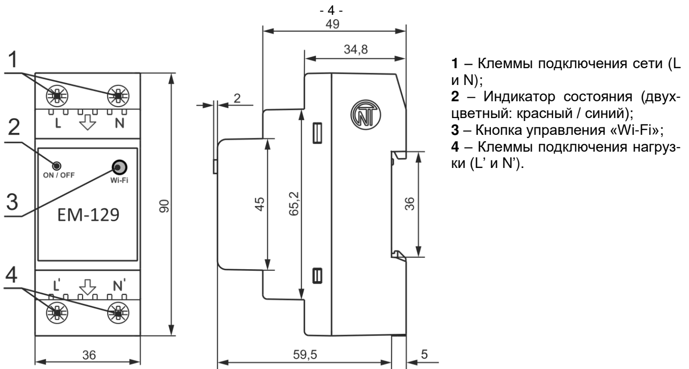
Рисунок 1 – Органы управления, габаритные и установочные размеры EM-129
