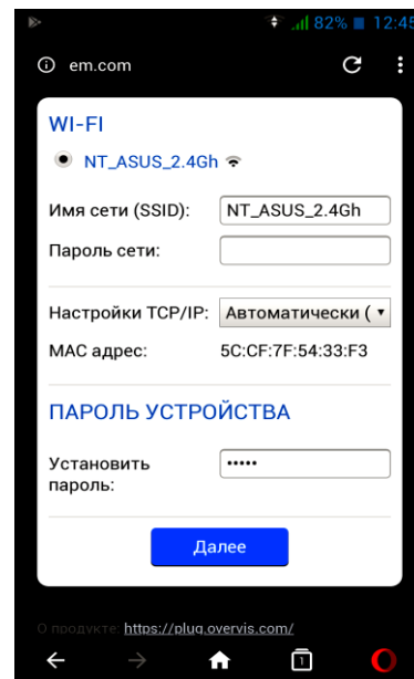
Рисунок 4 – Настройка Wi-Fi
