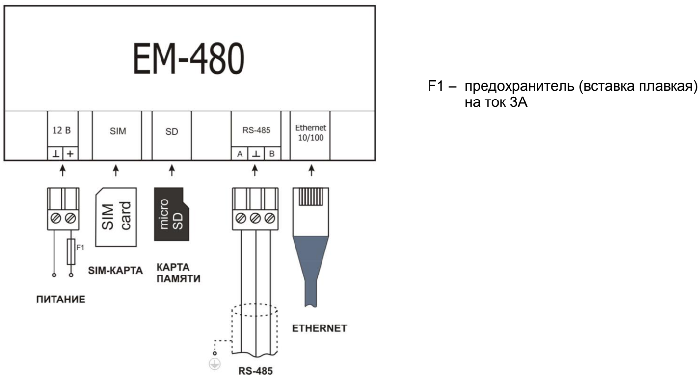
Рисунок 5.1 – Подключение изделия
