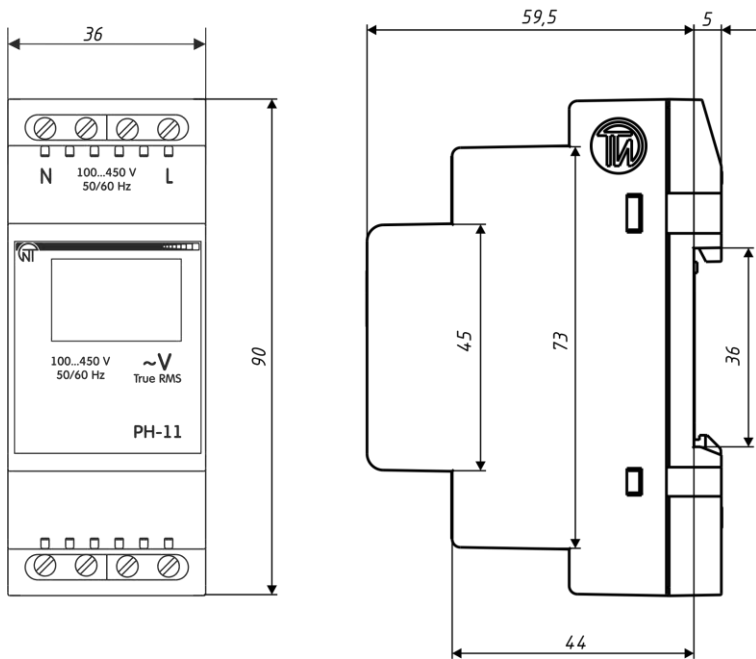
Рисунок 1 – Габаритные и установочные размеры РН-11
